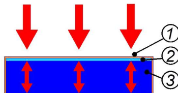
1 - Rivestimento in tessuto 2 - Lamina poliestere compatto 100 Kg/mc 3 - Poliestere densità 45-50 Kg/mc
